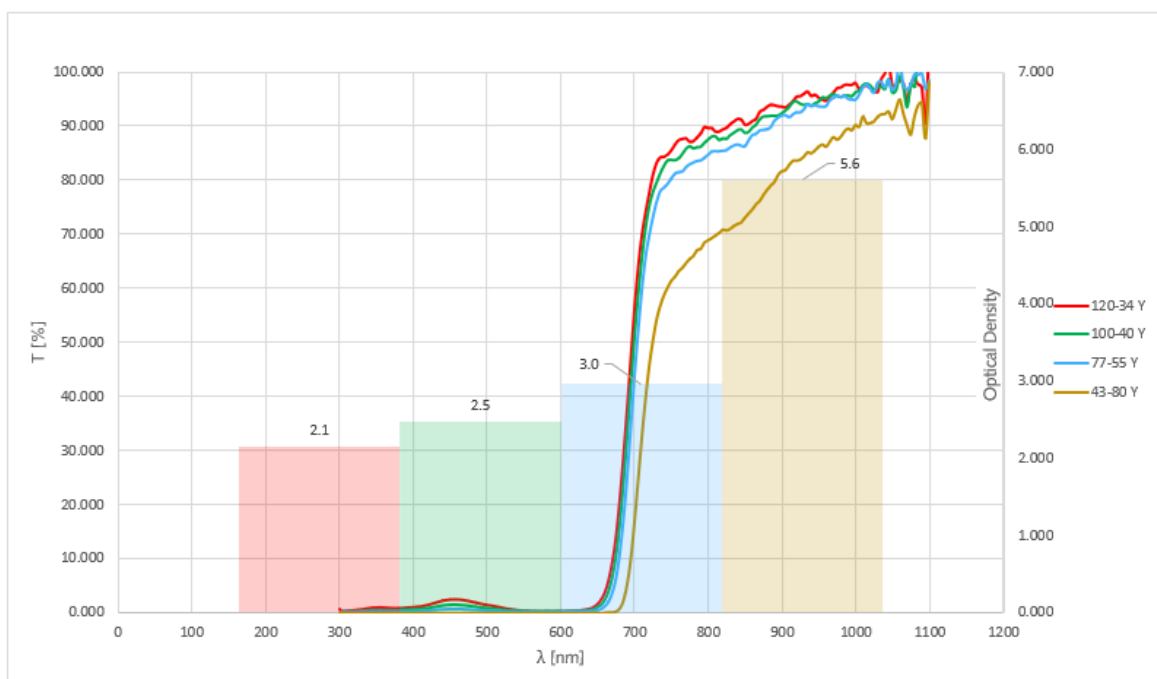
Figura 1: Opacidad alcanzada y transparencia a IR con diferentes mallas (barniz transparente + colorante 70:30 con un 3 % de Serie 600-HVA). La aplicación con una malla 43-80 Y no es adecuada para todos los sensores debido a la reducida transparencia a IR; sin embargo, puede ser útil para aplicaciones especiales (por ejemplo, curar un adhesivo sensible a IR a través de la capa de tinta).
